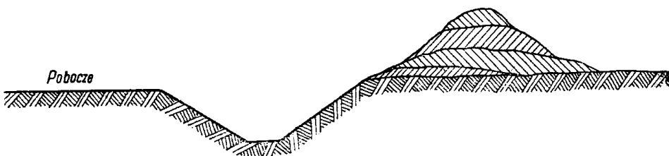
b) Niewłaściwe składanie namułu z oczyszczenia rowu tuż przy skarpie rowu (rów może być zamulony ponownie przez obsuwający się namuł)
