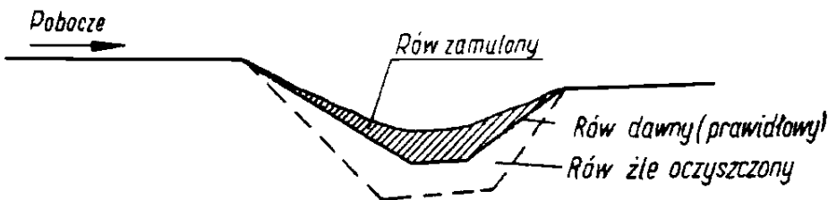
a) Niepotrzebne pogłębienie dna rowu przy usuwaniu namułu (mogą powstawać zastoiska wodne)
