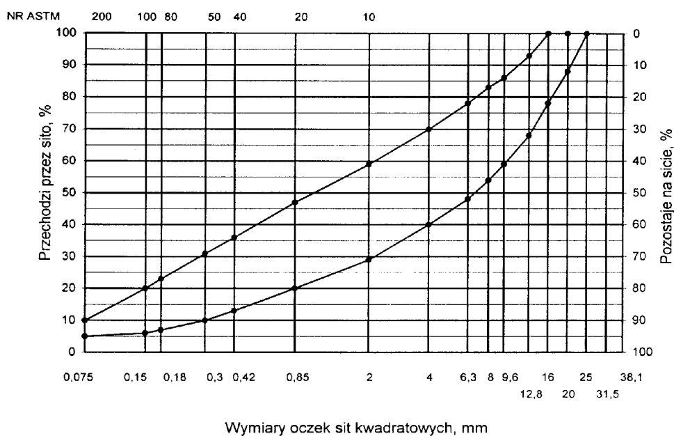
Rys. 1. Krzywe graniczne uziarnienia mieszanki mineralnej BA od 0 do 20 mm do warstwy ściernic nawierzchni drogi o obciążeniu ruchem dla KR1 lub KR2
